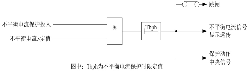
图 4-5 不平衡电流保护逻辑框图
