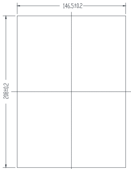
图 3-2 安装开孔尺寸
