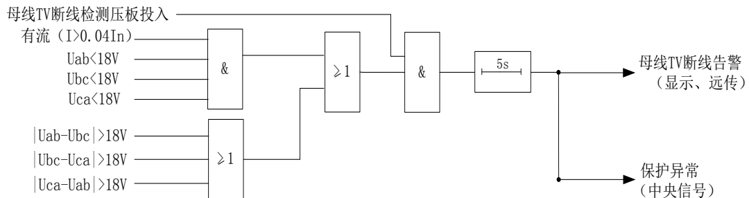
图 4-7 母线 TV 断线检测逻辑框图
