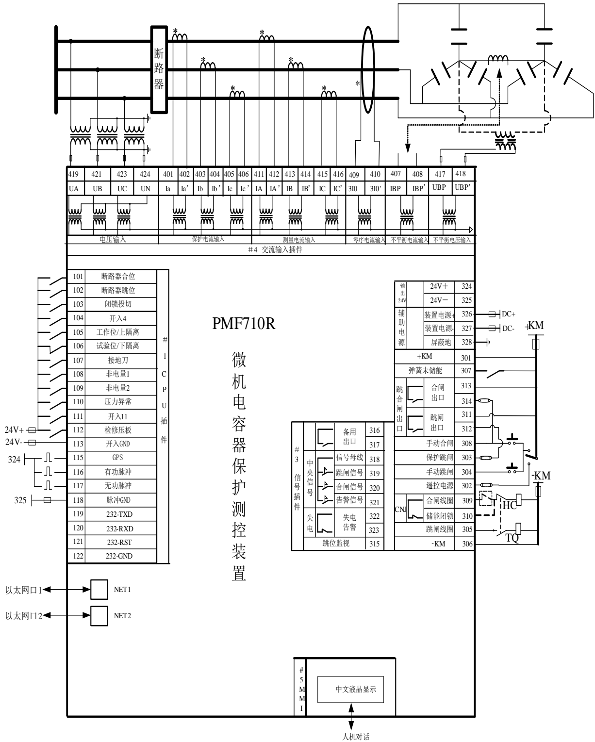
PMF710R-2NET 接线示意图
