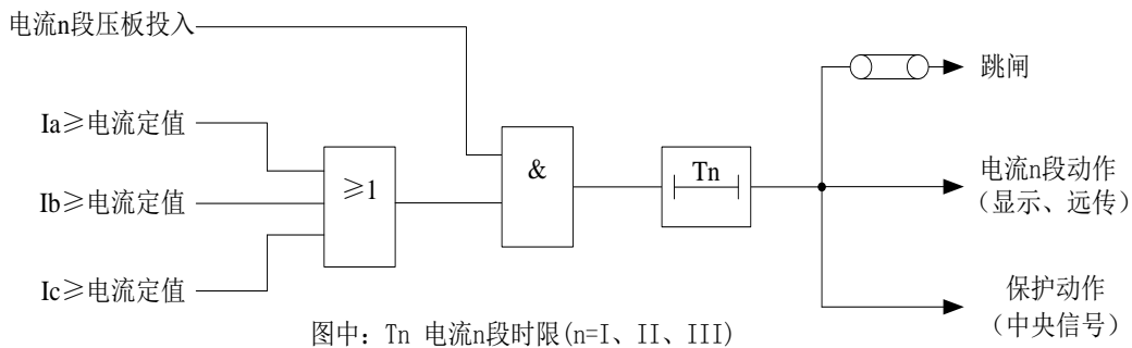
图 4-1 三段式电流保护逻辑框图
