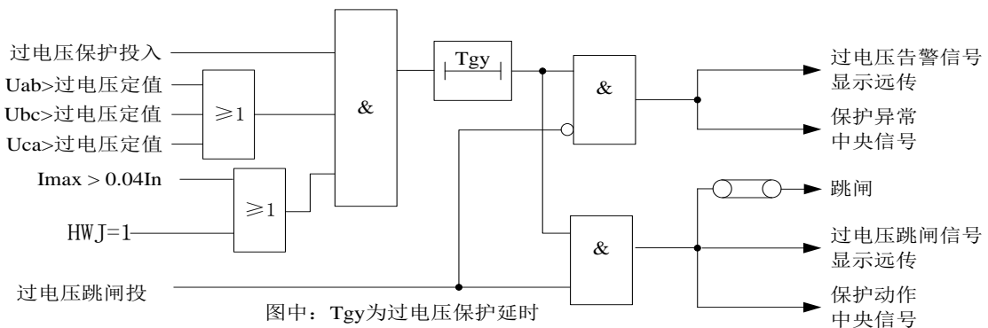
图 4-2 过电压保护逻辑框图
