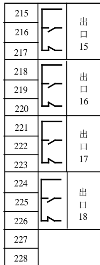
PMF710R-2NET 背部端子图 注: 备用出口默认配置闭锁投切
