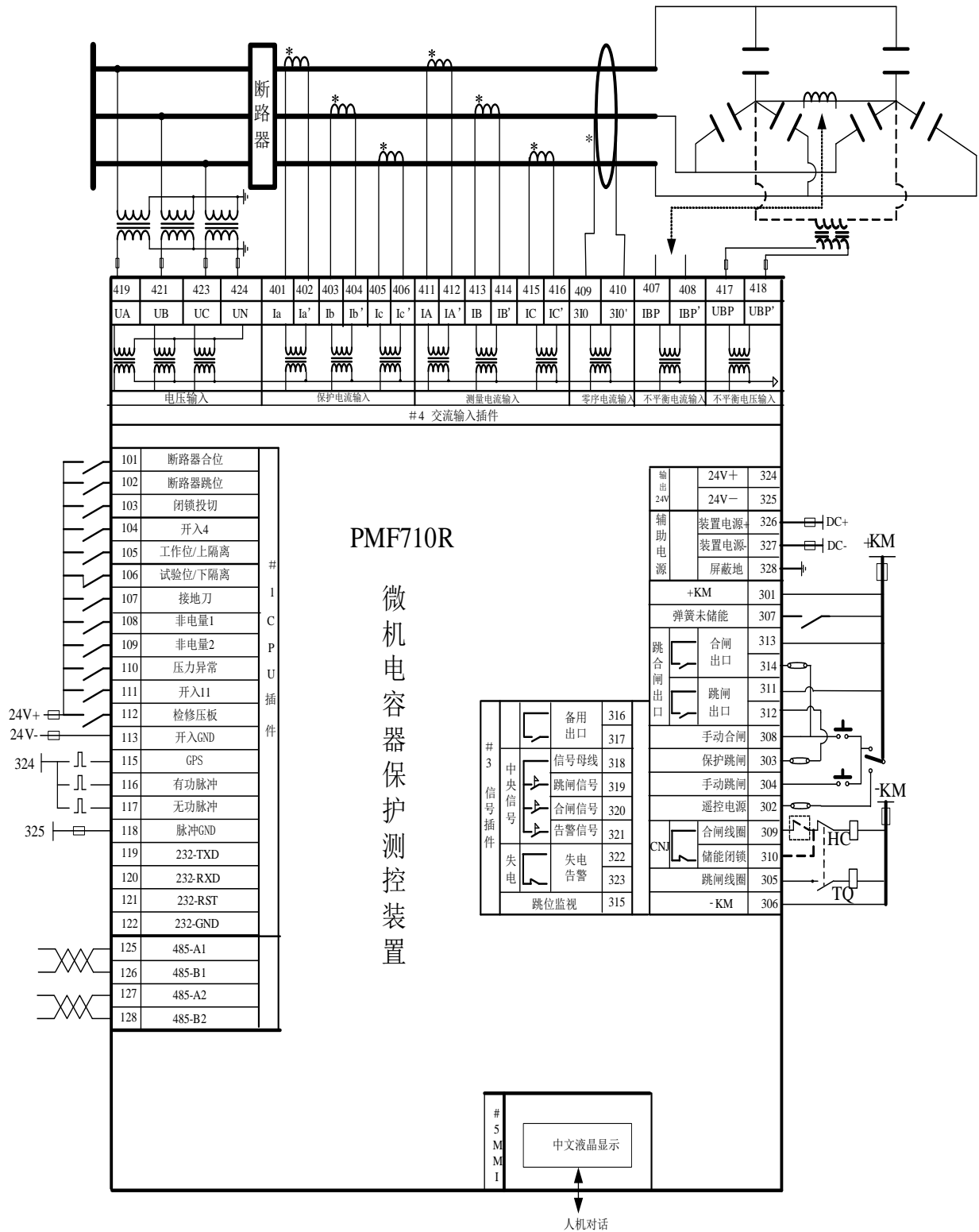
PMF710R-2RS485 接线示意图
